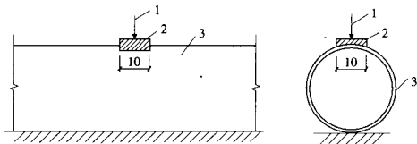
图 A. 0. 4 筒芯径向抗压荷载检验示意
