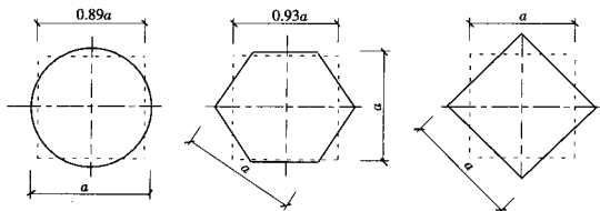
图4 支座等效宽度
