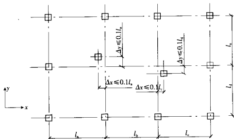
图2 柱子离相邻柱中心线的最大偏移
