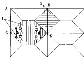
图 8 区格板中梁的从属面积
