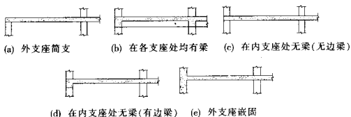
图5 计算板带端跨支座约束条件
